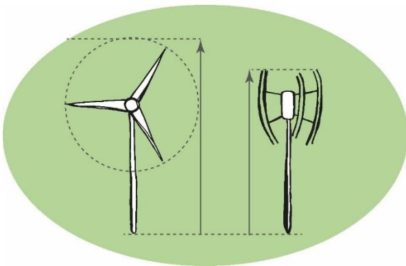
Afbeelding 2: Tiphoogte van een horizontale as-turbine (links) en verticale as-turbine (rechts)
